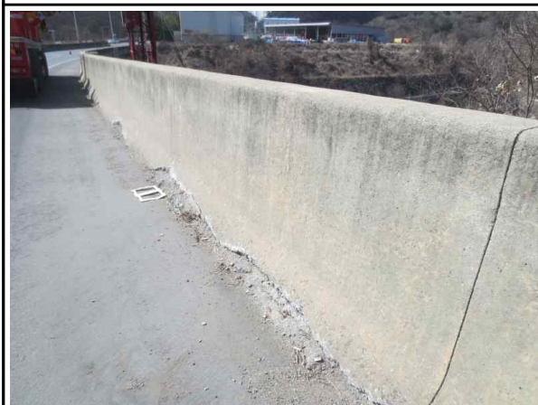
방호벽 전경
