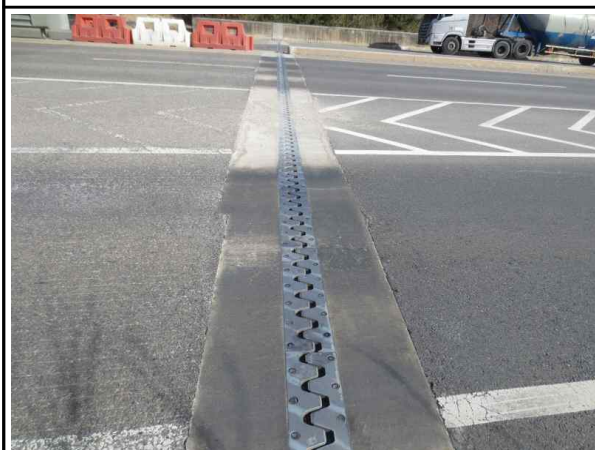
신축이음 전경
